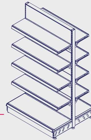
Gondola Unit / Çift Yönlü Orta Reyon H: 1850 mm L: 1000 mm 500B / 400 / 400 / 400 / 400 x 2
