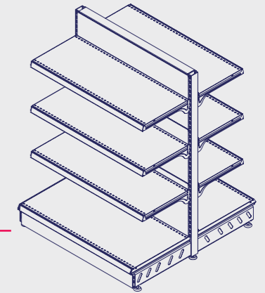
Gondola Unit / Çift Yönlü Orta Reyon H: 1430 mm L: 1000 mm 500B / 400 / 400 / 400 x 2
