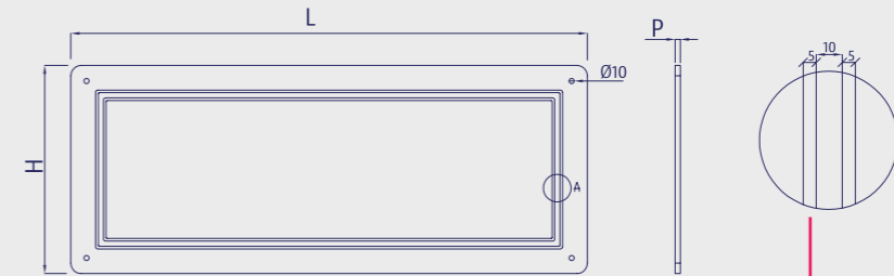
Channel Detail Kanal Detayı
